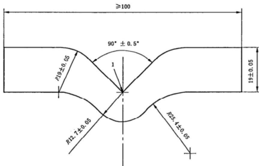
图 2 直角形试样裁刀所裁试样
